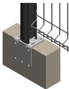
Platine équerre (ext.)
