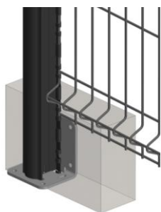
Platine anglaise (ext.)
